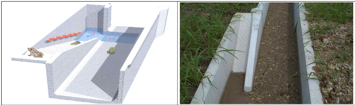
수로탈출시설(생태측구) 예시도
